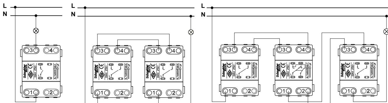
Еднополюсен ключ
