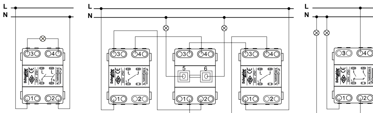
Двуполумен ключ
